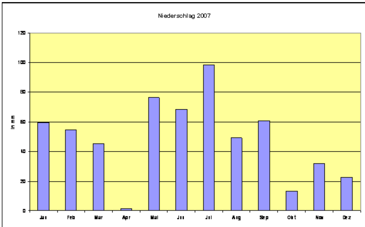
Temperatur und Niederschlag 2007 Klimastation am Nationalpark Unteres Odertal Gatow Forstrevier Wildbahn (Quelle: Nationalpark Unteres Odertal Jahresbericht 2007)
